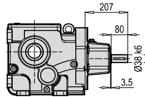
K 60390 DA W
