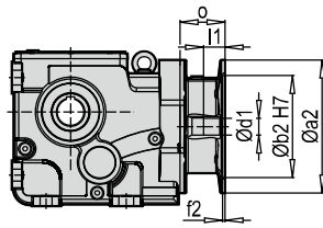
K 60390 DA PAM B5/B14
