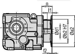
K 60390 DA/B14 PAM B5/B14
