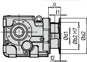
K 60390 DG/B14 PAM B5/B14
