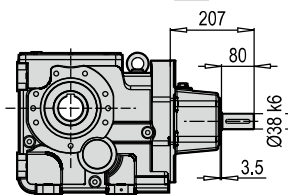
K 60390 DA/B14 W
