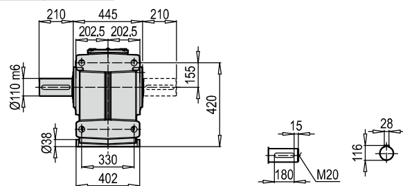
TMA - ÇMA / B14
