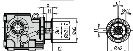
K 100390 DA/B14 PAM B5/B14
