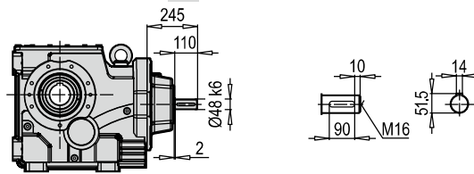
K 100390 DA/B14 W
