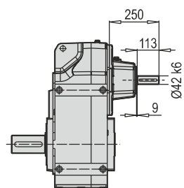
D/M 902 - 903 B5 W
