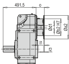
M 902 - 903 PAM B5/B14
