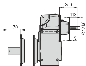
D/M 902 - 903 B5 W
