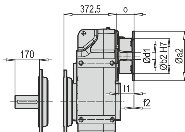
D/M 902 - 903 B5 PAM B5/B14
