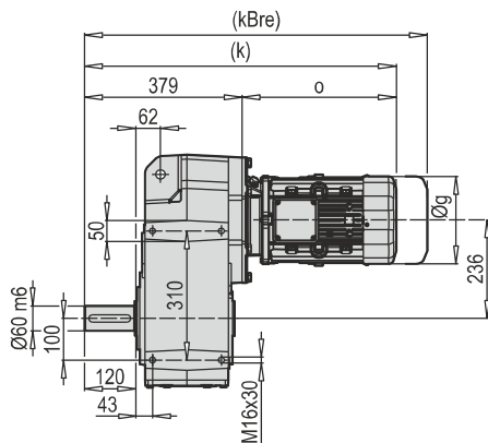
D/M 602 - 603 B5
