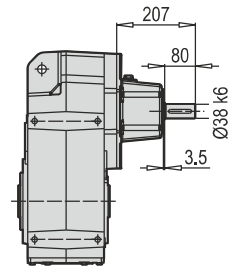
D 602 - 603 W
