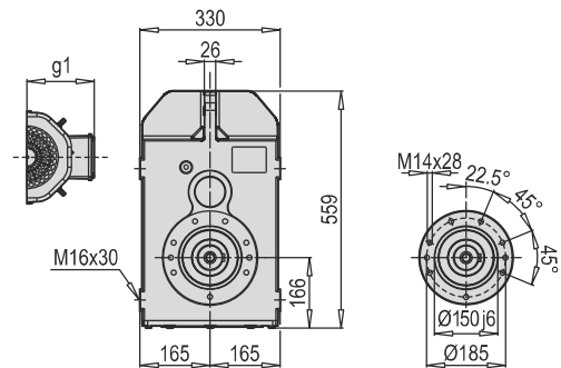
M 602 - 603 B14
