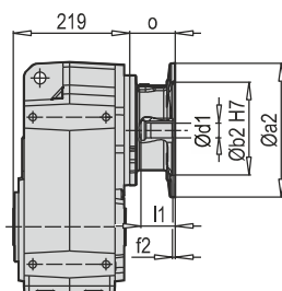
D 502 - 503 PAM B5/B14
