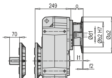
D/M 502 - 503 B5 PAM B5/B14
