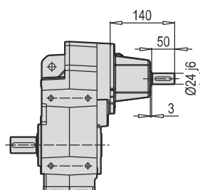
D/M 352 - 353 B5 W
