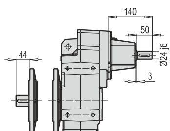
D/M 352 - 353 B5 W
