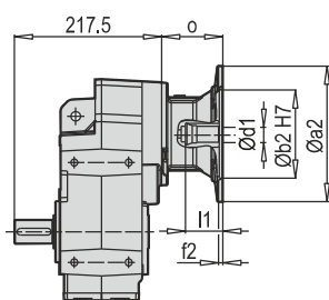
M 352 - 353 PAM B5/B14
