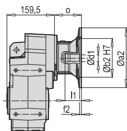
D 352 - 353 PAM B5/B14
