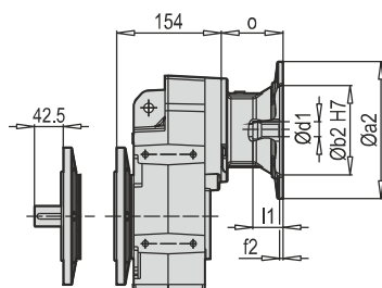
D/M 302 - 303 B5 PAM B5/B14
