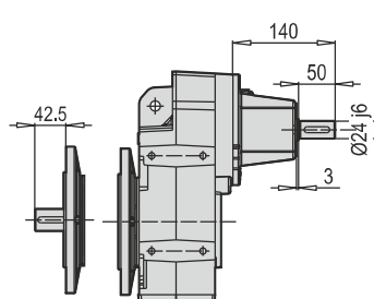
D/M 302 - 303 B5 W
