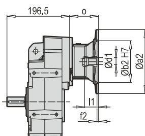
M 302 - 303 PAM B5/B14
