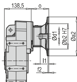
D 302 - 303 PAM B5/B14
